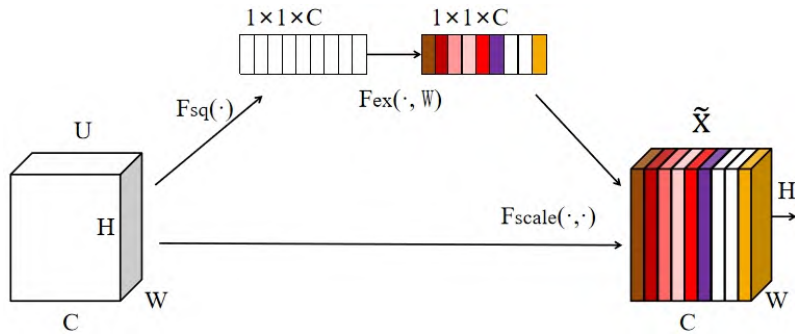
图 11 SE 注意力机制架构示意图 Fig.11 Architecture of the SE attention mechanism
